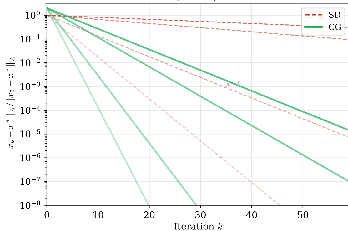
Error bound \|x_k - x^*\|_A vs. iteration
